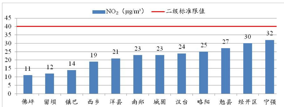
图 18 2023 年 1~3 月各县区 NO 2 浓度及达标情况
