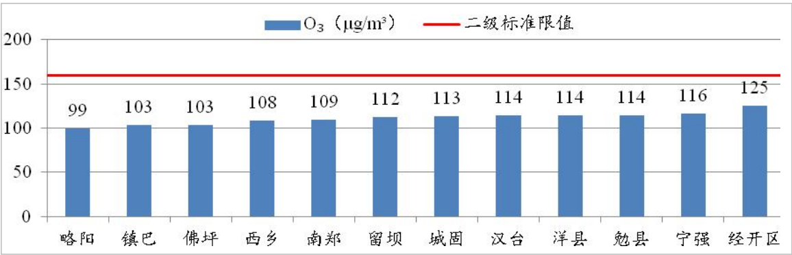
图 10 2023 年 3 月各县区 O 3 浓度及达标情况
