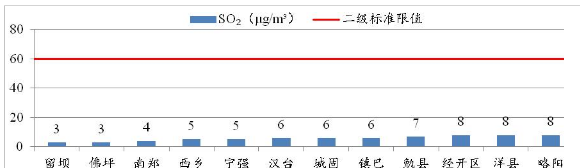
图7 2023年3月各县区SO 2 浓度及达标情况
