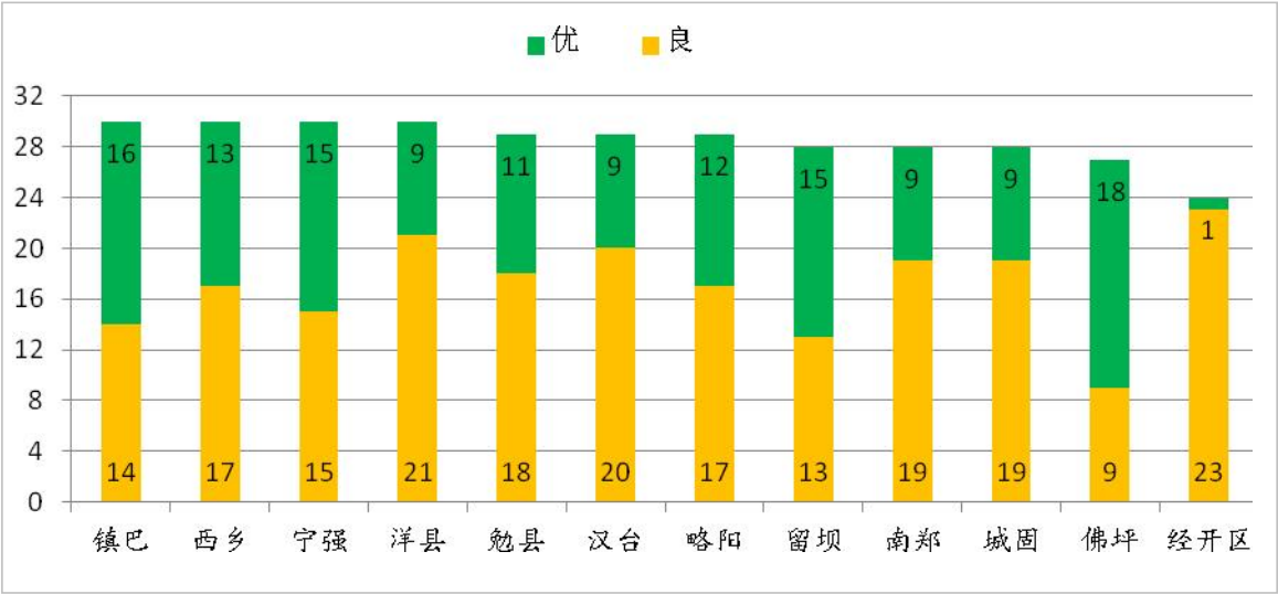
图 1 2023 年 3 月各县区环境空气质量优良天数图（单位：天）
