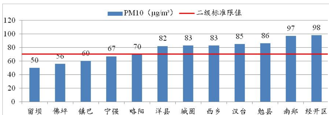
图 15 2023 年 1~3 月各县区 pM 10 浓度及达标情况
