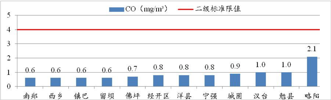
图 9 2023 年 3 月各县区 CO 浓度及达标情况
