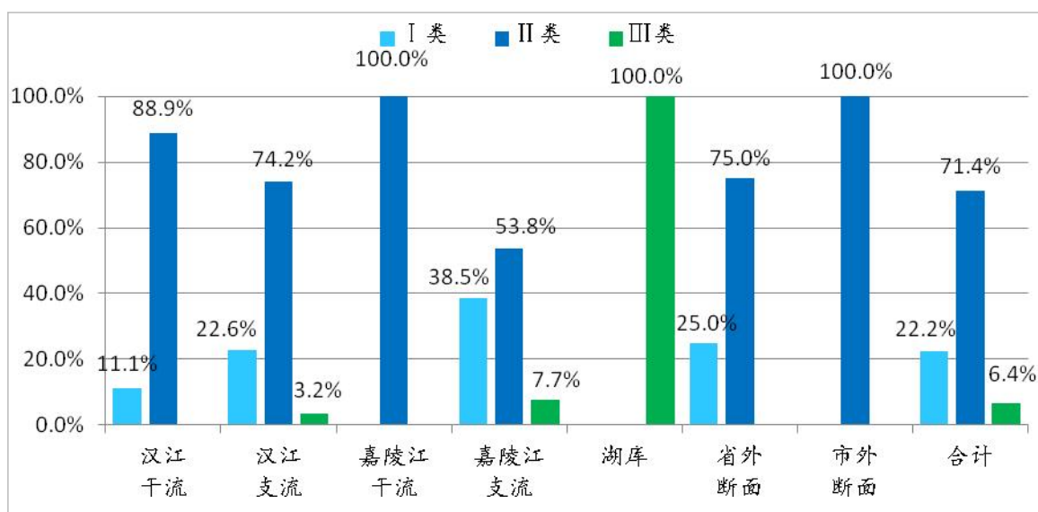
图 21 2023 年 3 月全市地表水断面水质类别比例图
