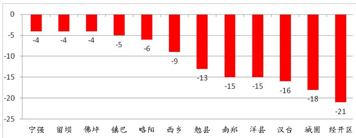
图 12 2023 年 1~3 月县区环境空气质量优良天数较去年同比变化情况（单位：天）
