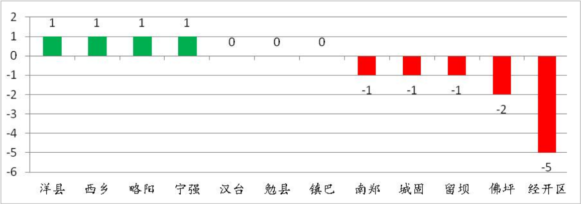
图 2 2023 年 3 月各县区环境空气质量优良天数较去年同比变化情况（单位：天）
