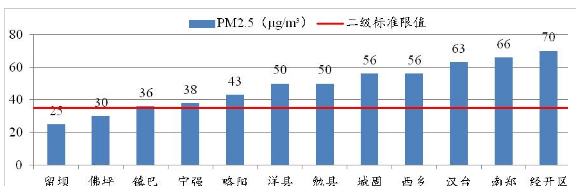
图 16 2023 年 1~3 月各县区 pM 2.5 浓度及达标情况
