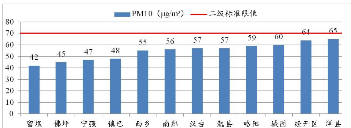
图5 2023年3月各县区pM 10 浓度及达标情况
