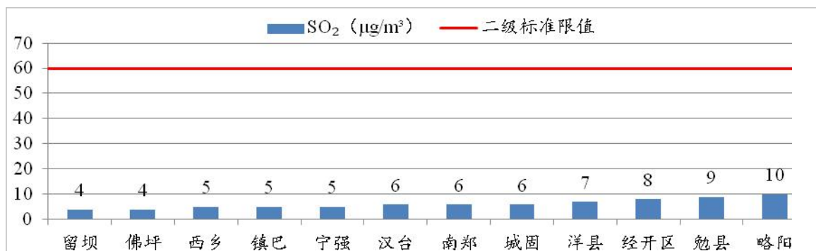
图 17 2023 年 1~3 月各县区 SO 2 浓度及达标情况
