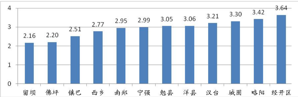
图 3 2023 年 3 月各县区环境空气质量综合指数
