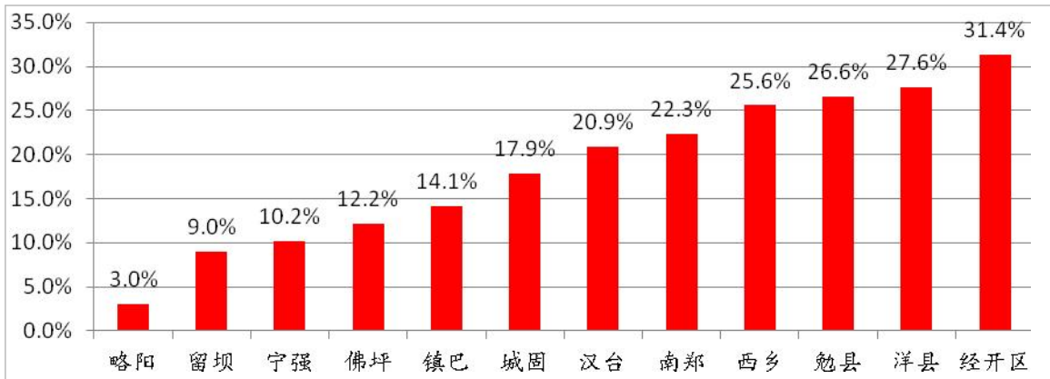
图 14 2023 年 1~3 月县区环境空气质量综合指数较去年同比变化情况
