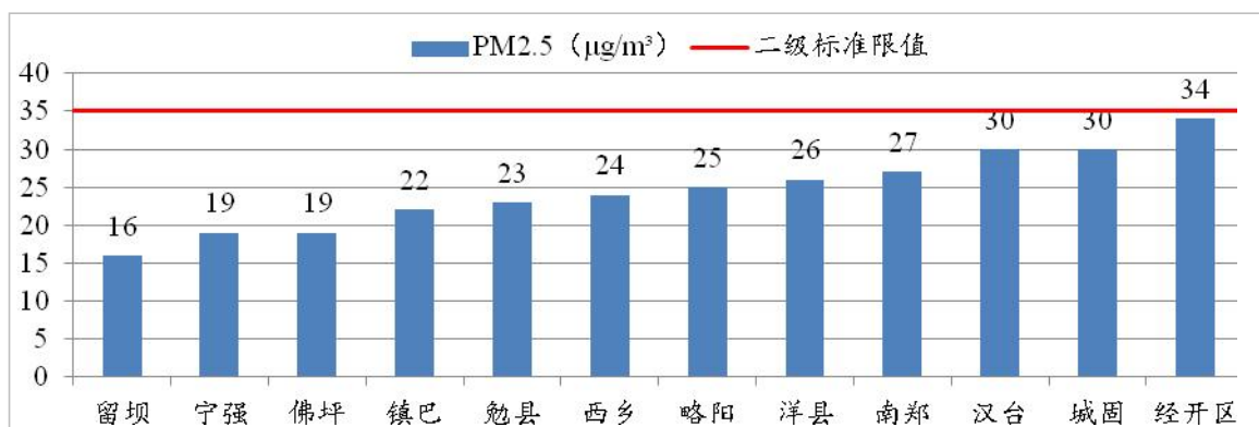
图6 2023年3月各县区PM 2.5 浓度及达标情况
