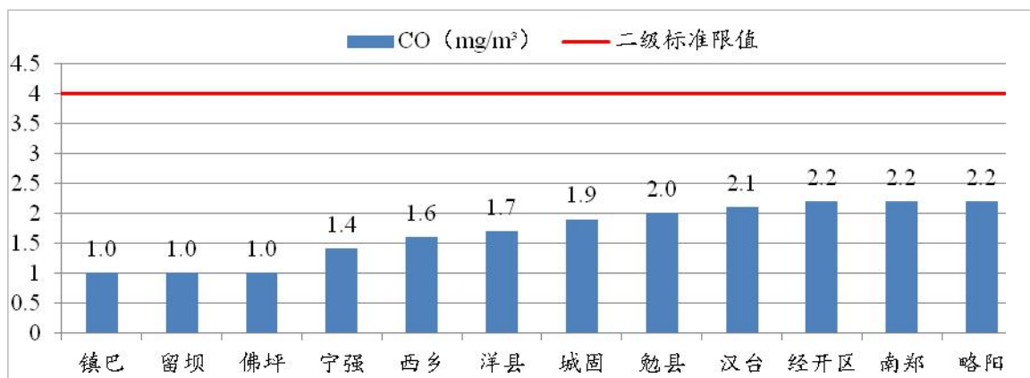
图 19 2023 年 1~3 月各县区 CO 浓度及达标情况
