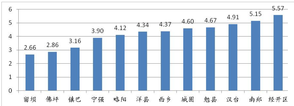
图 13 2023 年 1~3 月县区环境空气质量综合指数
