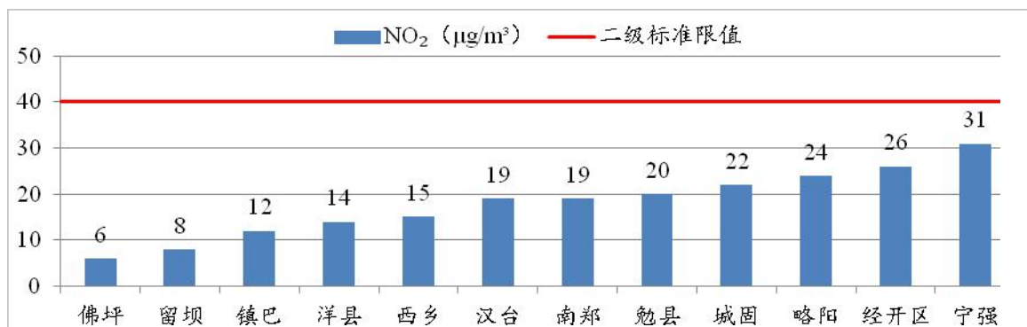
图8 2023年3月各县区NO 2 浓度及达标情况
