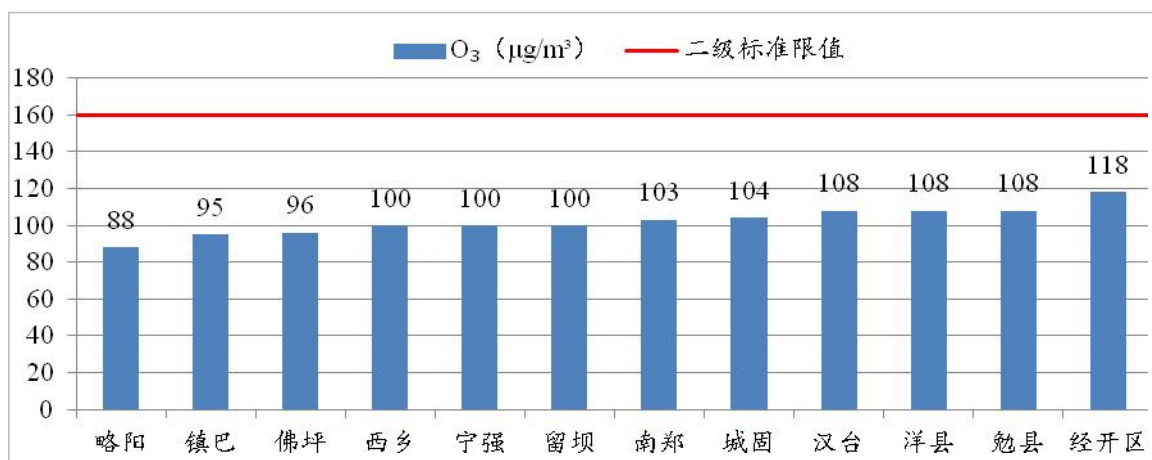
图 20 2023 年 1~3 月各县区 O_3 浓度及达标情况
