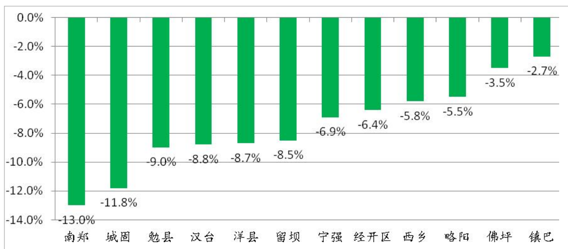
图4 2023年3月各县区环境空气质量综合指数较去年同比变化情况
