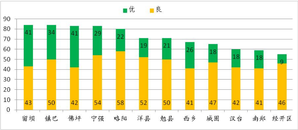
图 11 2023 年 1~3 月县区环境空气质量优良天数（单位：天）
