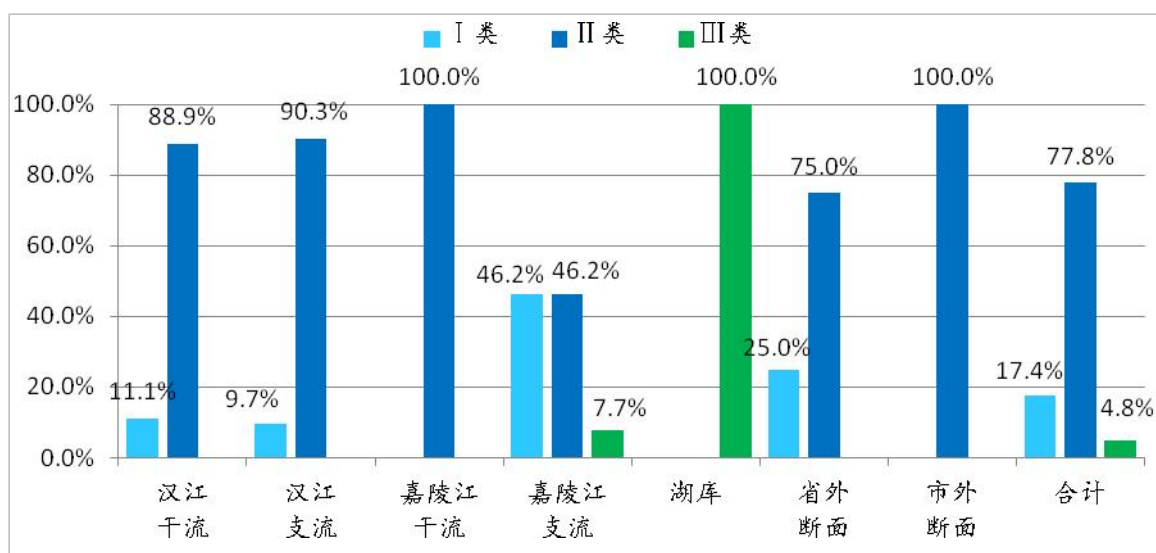
图 22 2023 年 1~3 月全市地表水断面水质类别比例图
