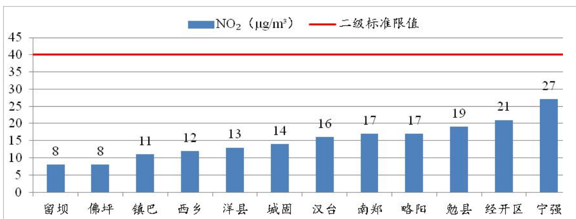
图 18 2023 年 1~8 月各县区 NO 2 浓度及达标情况
