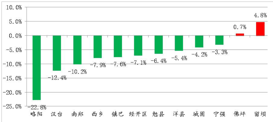
图4 2023年8月各县区环境空气质量综合指数较去年同比变化情况
