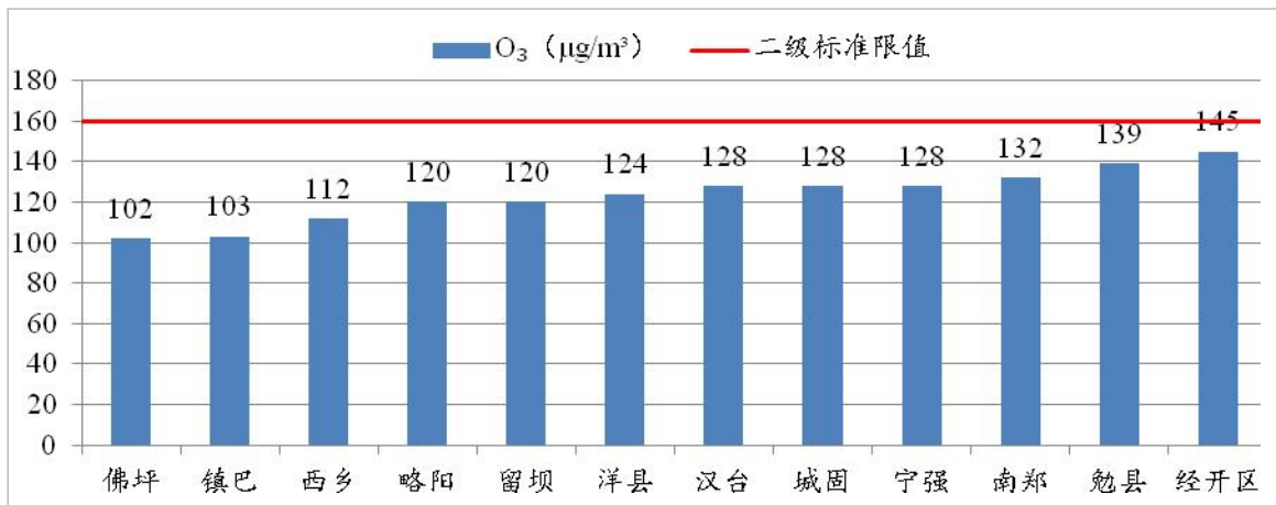
图 20 2023 年 1~8 月各县区 O 3 浓度及达标情况
