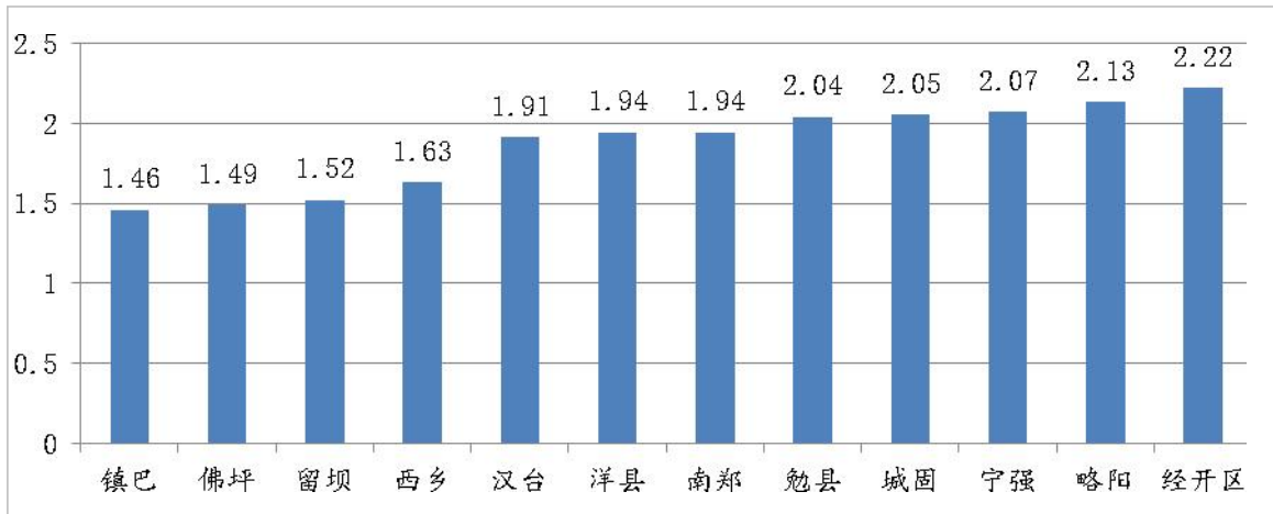
图3 2023年8月各县区环境空气质量综合指数
