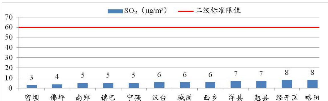
图 17 2023 年 1~8 月各县区 SO 2 浓度及达标情况
