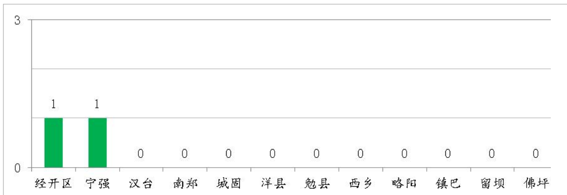
图2 2023年8月各县区环境空气质量优良天数较去年同比变化情况(单位:天)
