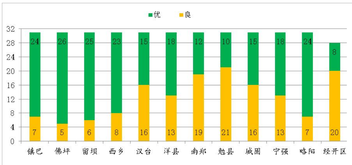
图1 2023年8月各县区环境空气质量优良天数图(单位:天)
