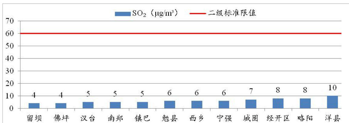
图7 2023年8月各县区SO 2 浓度及达标情况
