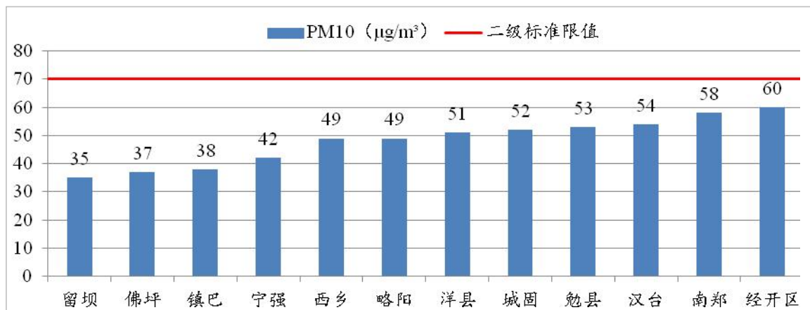
图 15 2023 年 1~8 月各县区 pM 10 浓度及达标情况
