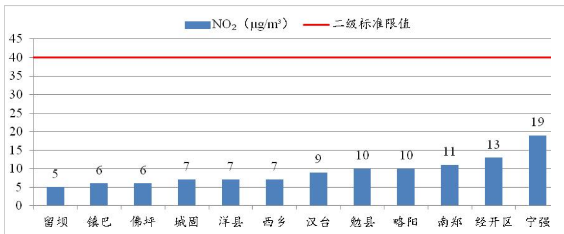
图8 2023年8月各县区NO 2 浓度及达标情况
