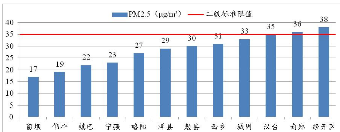
图 16 2023 年 1~8 月各县区 pM 2.5 浓度及达标情况
