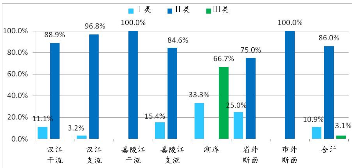
图 22 2023 年 1~8 月全市地表水断面水质类别比例图
