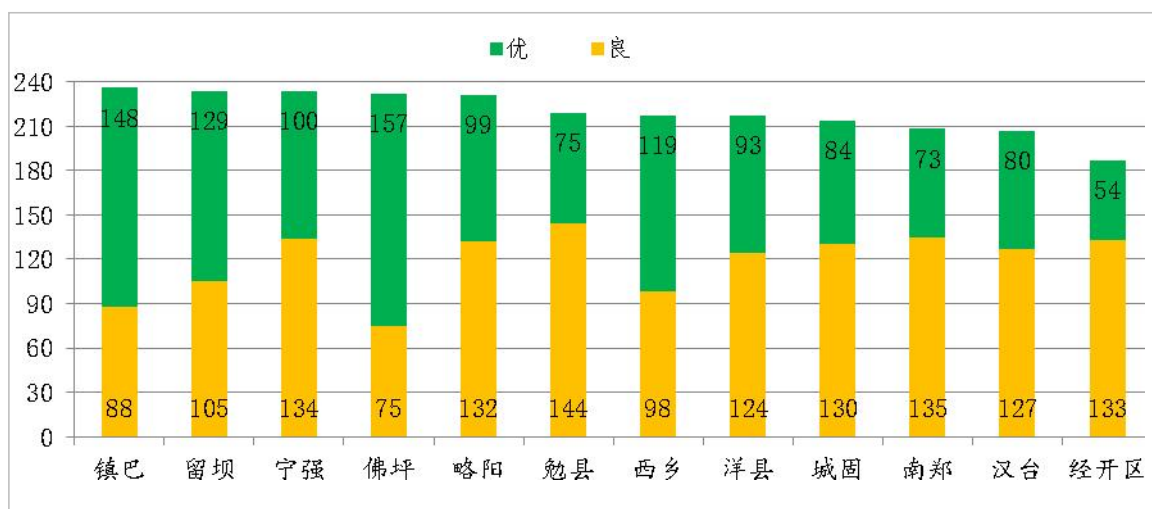
图 11 2023 年 1~8 月县区环境空气质量优良天数(单位: 天)
