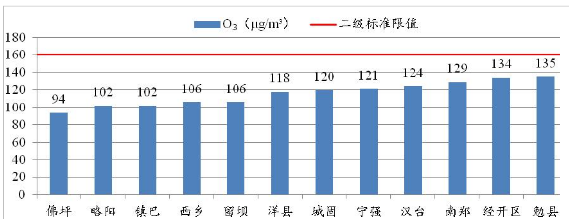
图10 2023年8月各县区O 3 浓度及达标情况
