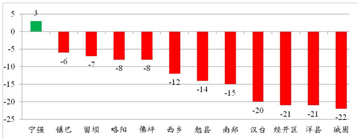
图 12 2023 年 1~8 月县区环境空气质量优良天数较去年同比变化情况 (单位: 天)
