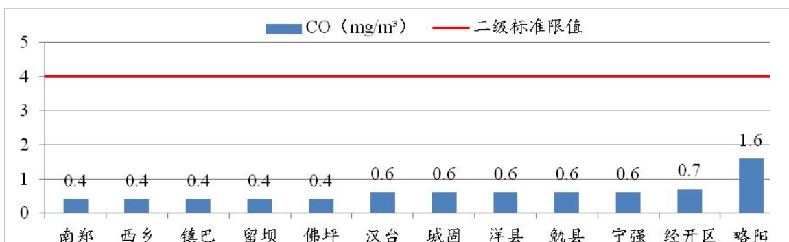
图9 2023年8月各县区CO浓度及达标情况
