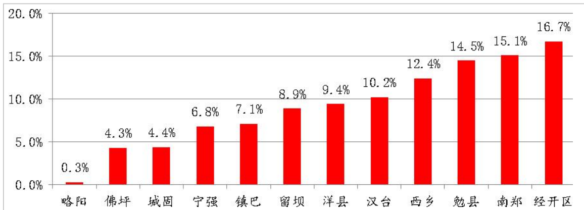
图 14 2023 年 1~8 月县区环境空气质量综合指数较去年同比变化情况
