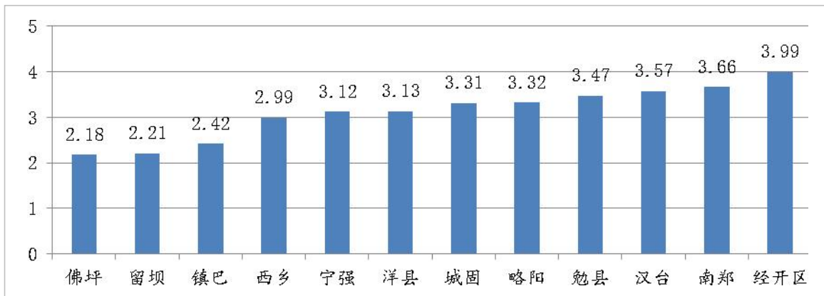
图 13 2023 年 1~8 月县区环境空气质量综合指数
