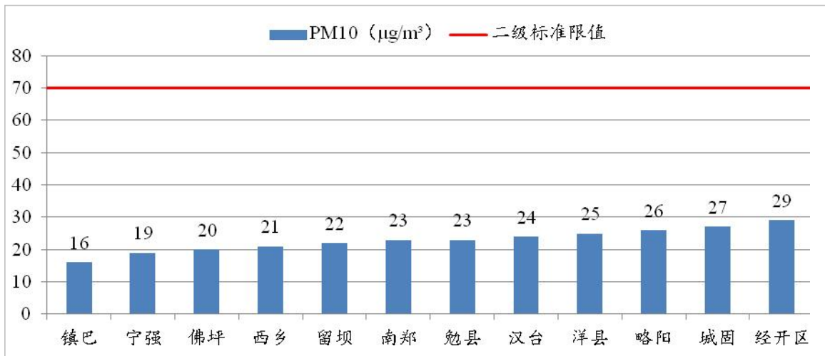
图5 2023年8月各县区 pM 10 浓度及达标情况
