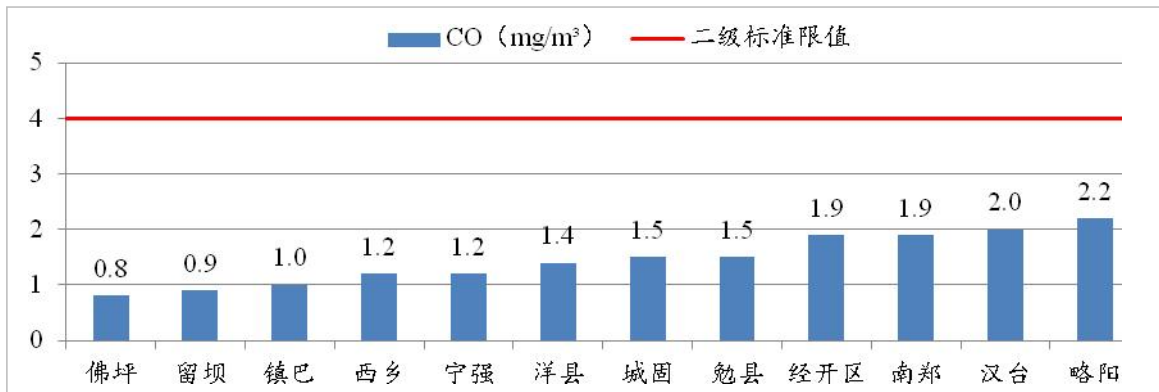
图 19 2023 年 1~8 月各县区 CO 浓度及达标情况
