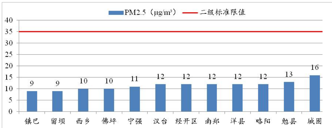
图6 2023年8月各县区 pM 2.5 浓度及达标情况
