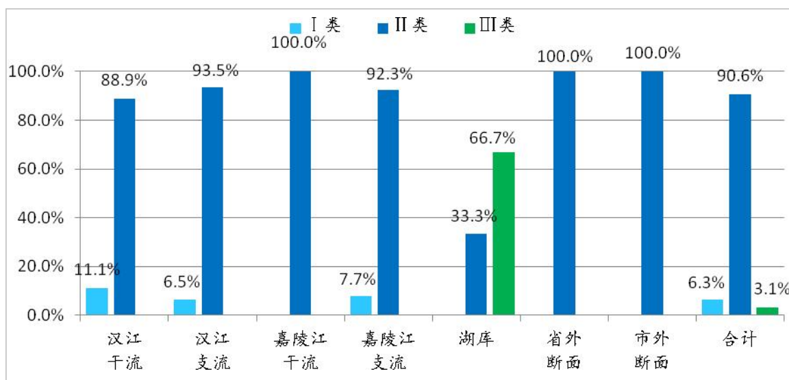
图 21 2023 年 8 月全市地表水断面水质类别比例图
